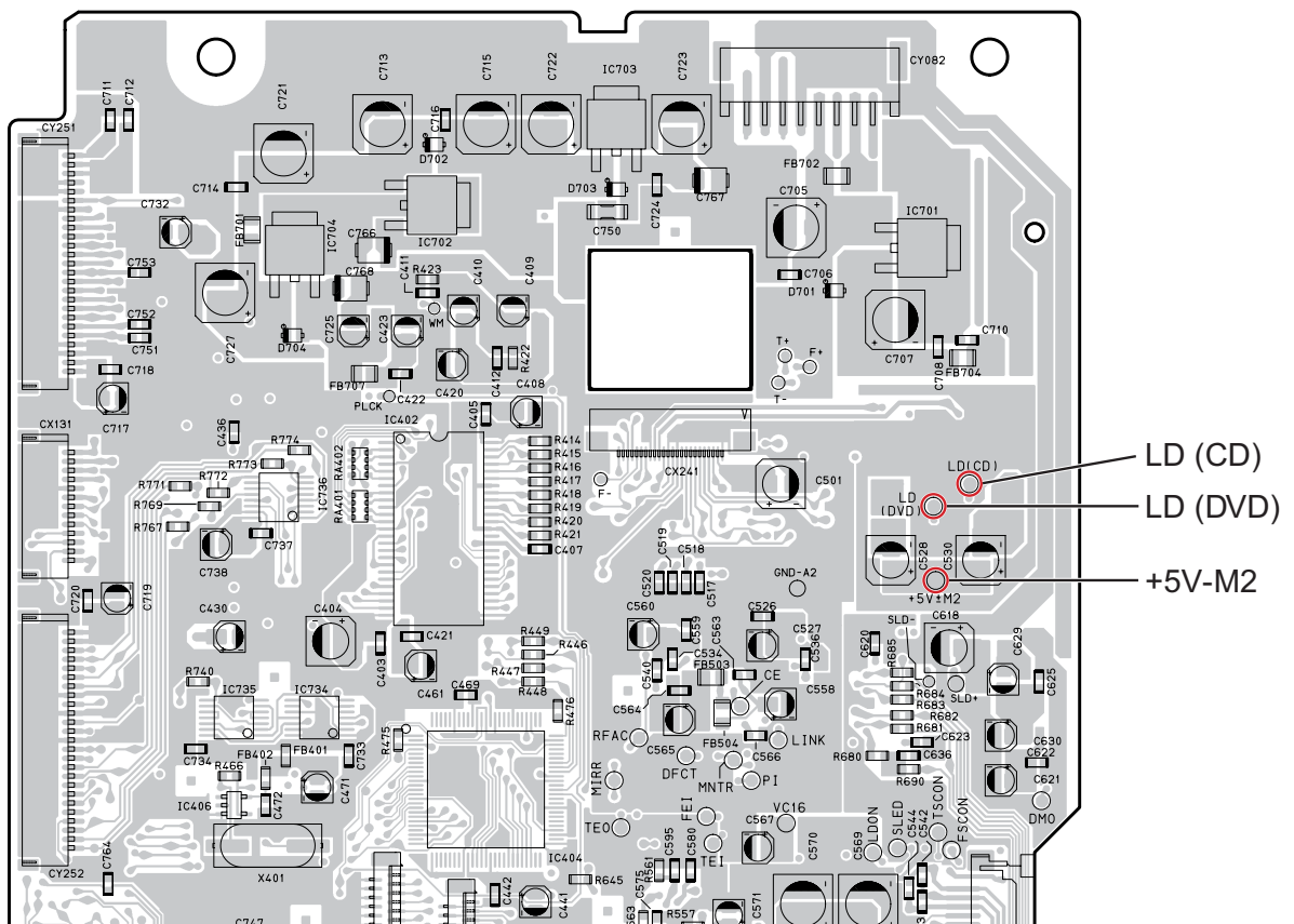
1U-3562 SACD MODULE P.W.B. unit foil side
