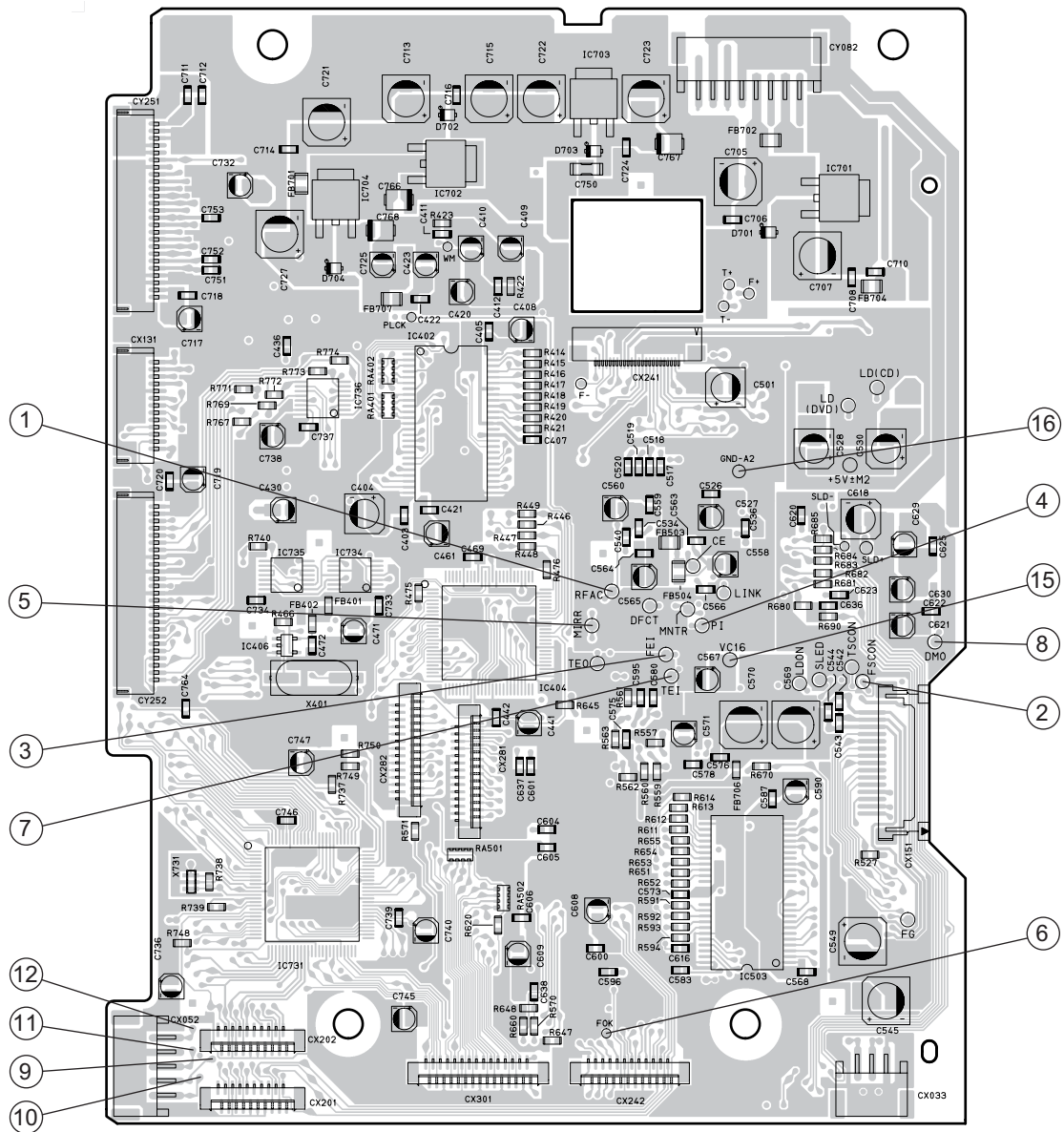
1U-3562 SACD MODULE P.W.B. unit foil side
