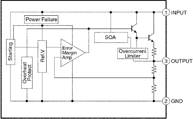
IC752 : C0CBCBG00012
