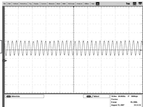
MT8520 DDR2_A_CLK0
