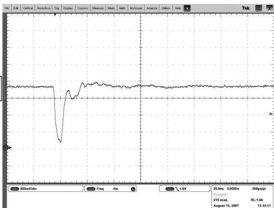
MT8520 DDR2_A_WE#
